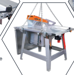
4 ausklappbare Kranösen
